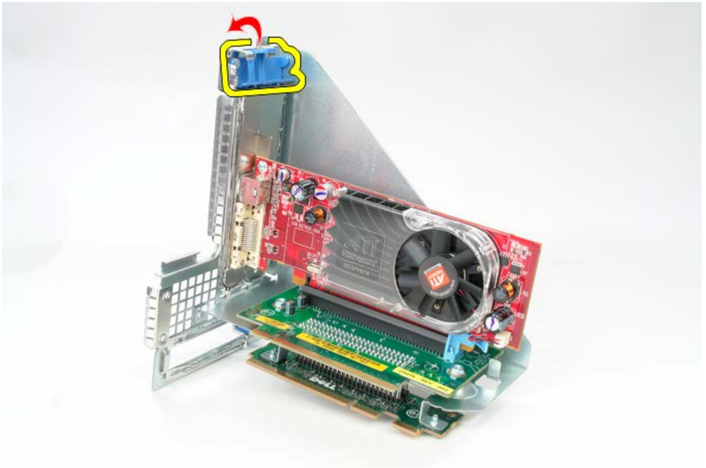
1 11 轻轻拉动提升板上的插卡释放门锁，将其脱离插卡并轻轻地将插卡从连接器中取出。
