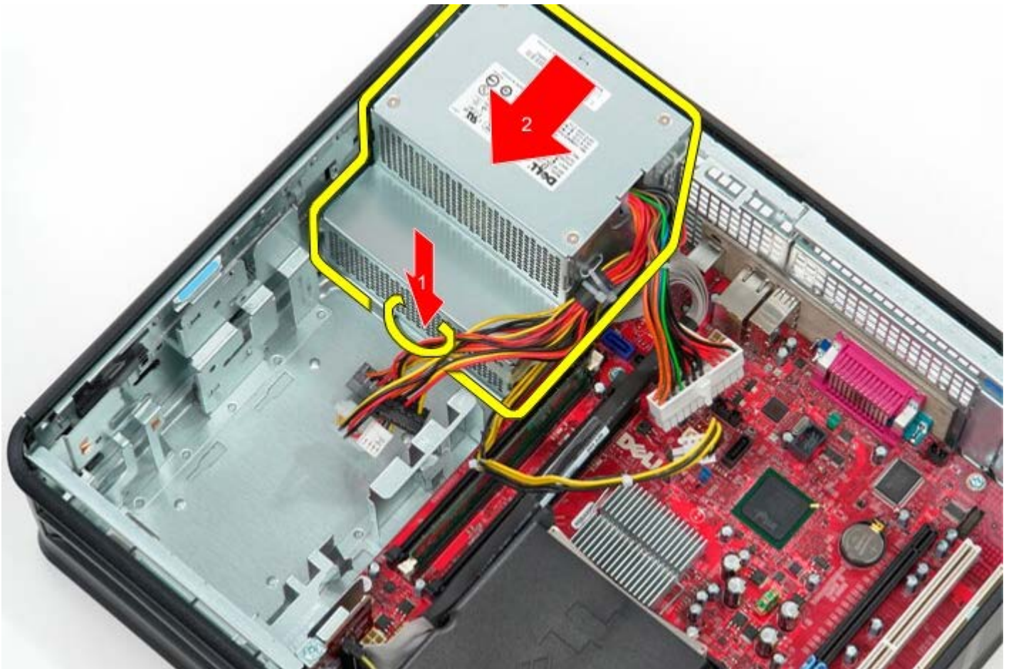
1 1 11 向上提起电源设备，将其从计算机中取出。
