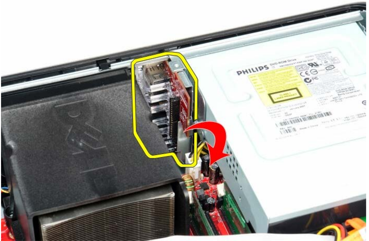
1 11 轻轻旋转 IO 面板，使其脱离计算机，然后从计算机卸下。
