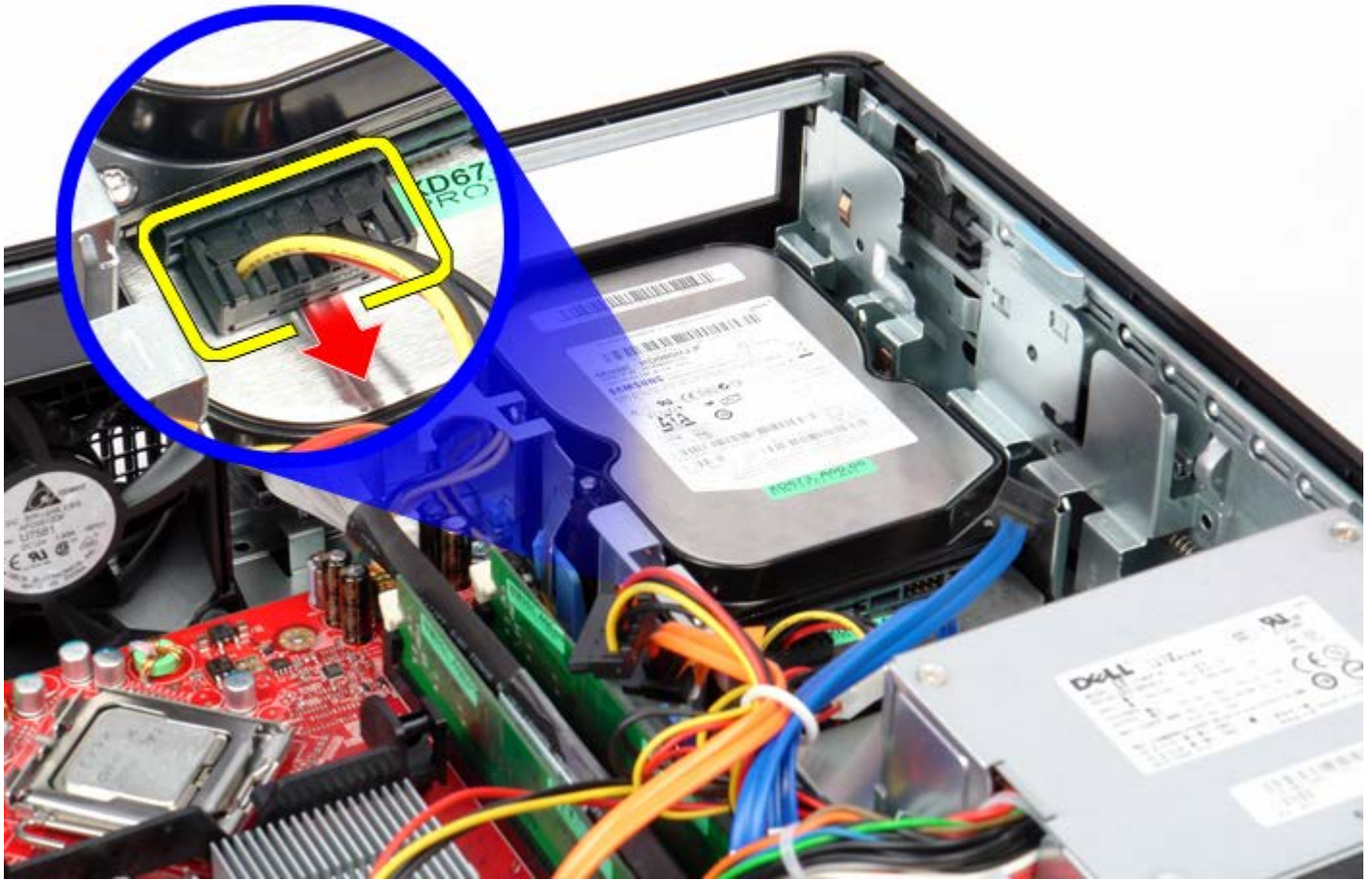
1 11 向上拉动释放门锁，并朝计算机背面滑动硬盘驱动器。
