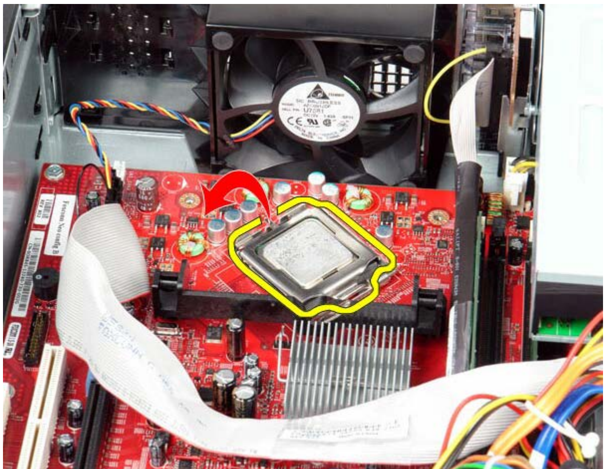
1 11 从计算机中卸下处理器。
