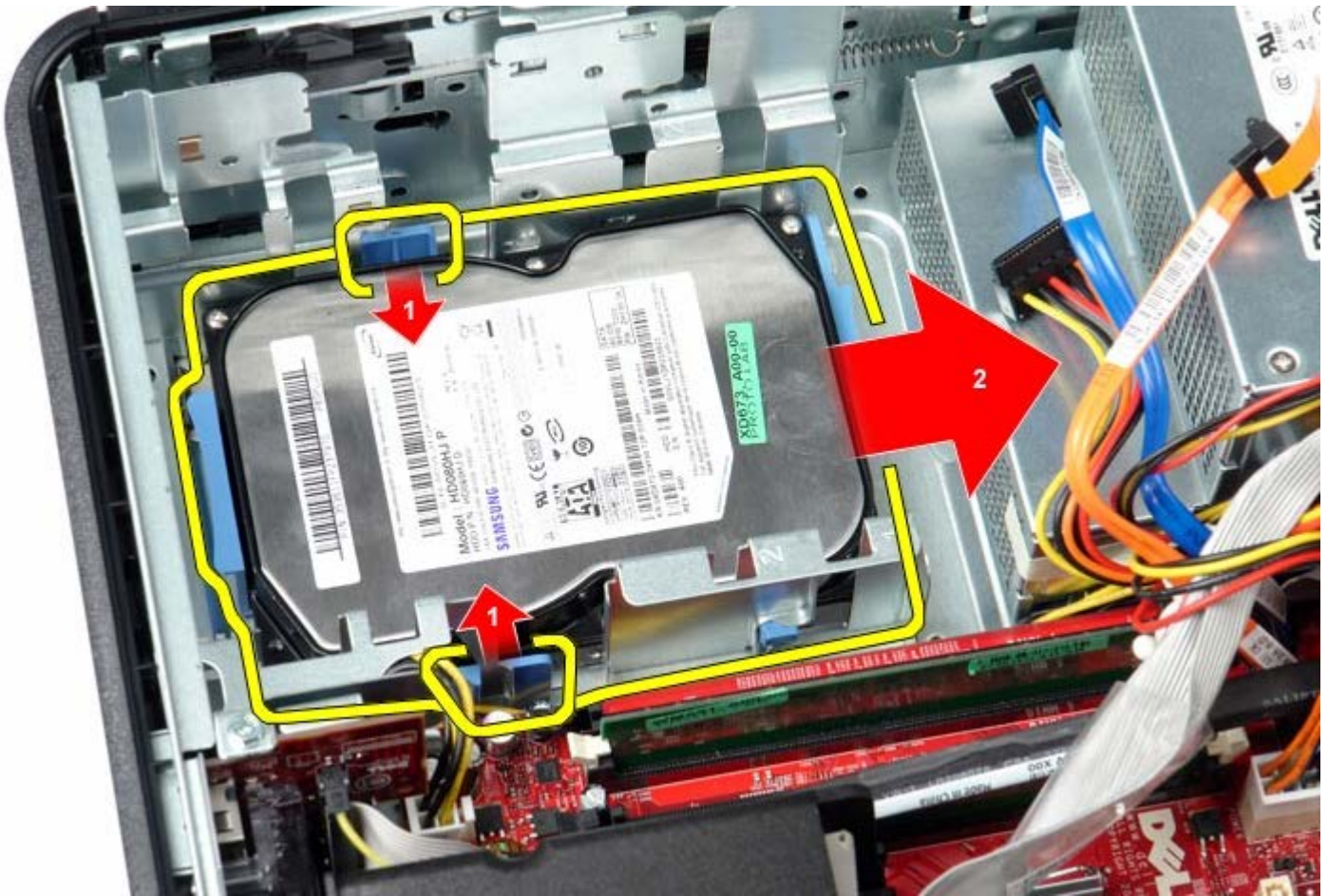
1 11 提起硬盘驱动器，将其从计算机中卸下。
