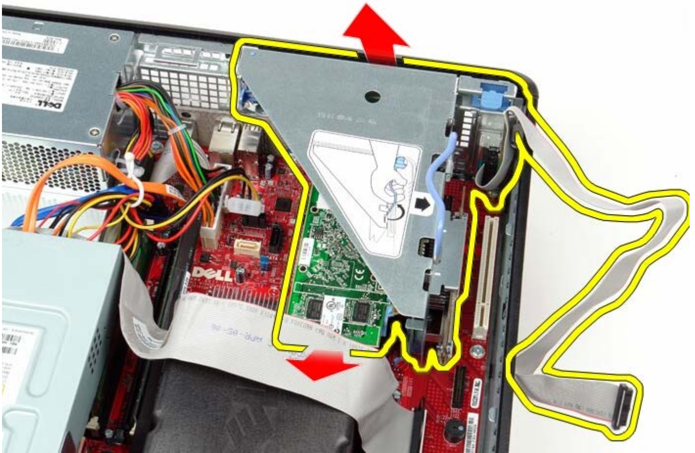
1 11 在提升卡固定框架上，向上旋转插卡固定门锁。
