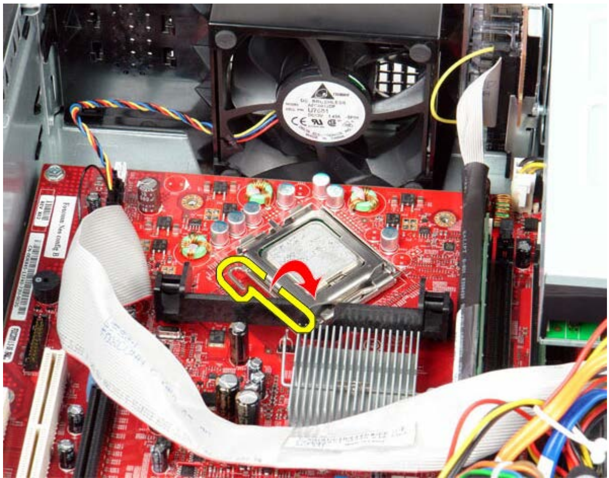
1 11 提起处理器护盖。
