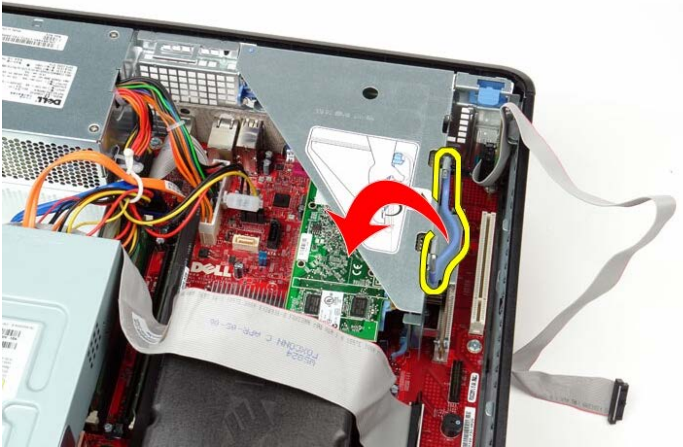
1 11 轻轻拉动提升卡固定框架手柄并向上提起提升卡固定框架，将其从计算机中取出。
